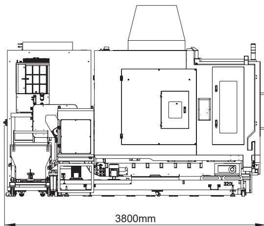
左视图
