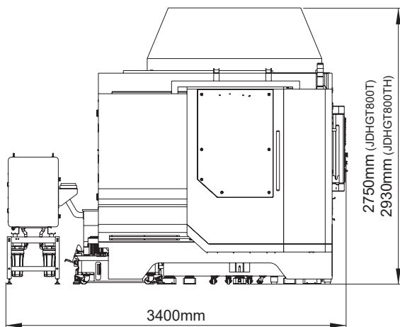
前视图
